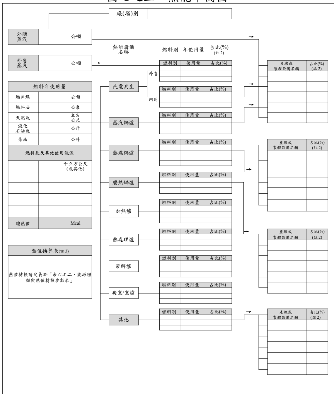
圖七之三、熱能平衡圖
